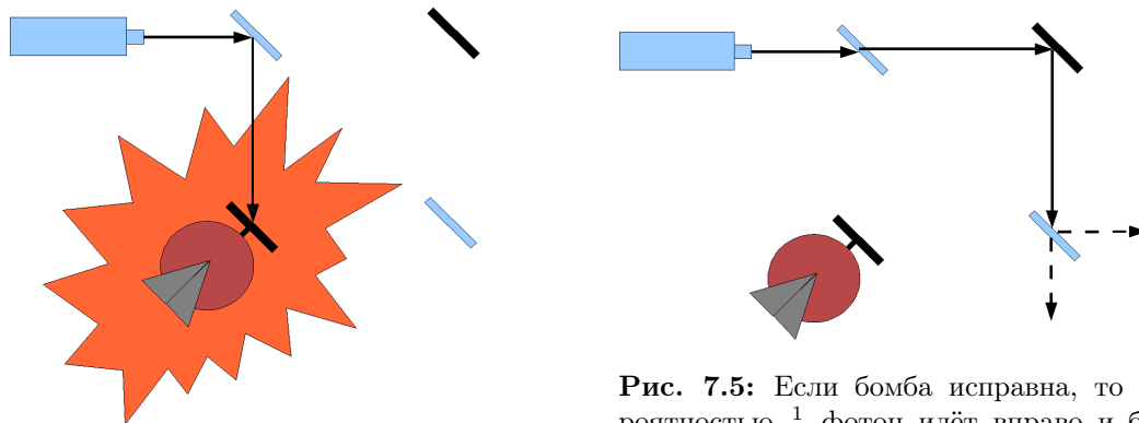
Рис. 7.4: Если бомба исправна, то с вероятностью \frac{1}{2} фотон идёт вниз и бомба взрывается.
