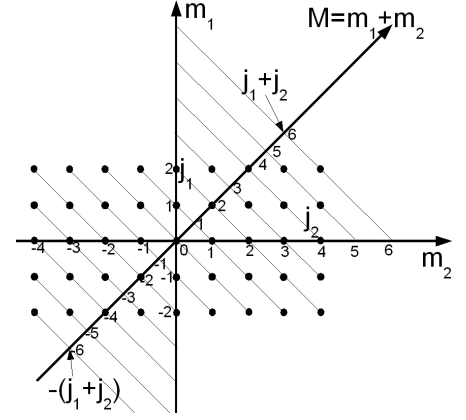
Рис. 15.4: Связь M с m_1 и m_2 .
