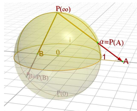
Рис. 15.2: Проекция комплексной плоскости на сферу Римана. Вид снизу в зеркальном отражении.
