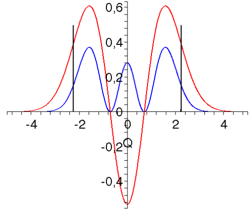
Рис. 12.4: Второе возбуждённое состояние гармонического осциллятора: \psi_2(Q) и |\psi_2(Q)|^2 .
