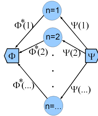
Рис. 3.5: Переход от \Psi в \Phi совершается через все возможные взаимоисключающие состояния n по стрелкам с соответствующими амплитудами согласно (3.13).
