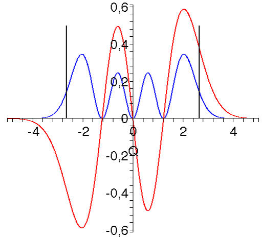
Рис. 12.5: Третье возбуждённое состояние: \psi_3(Q) и |\psi_3(Q)|^2 .
